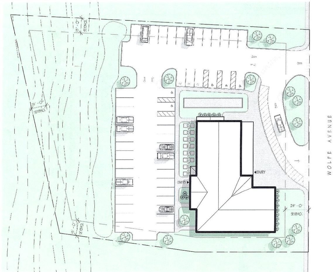
Site Plan 0 10 30
